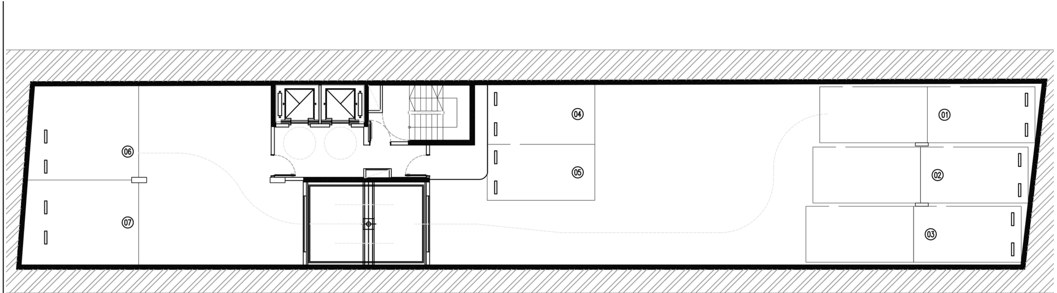
2do SUBSUELO (10 cocheras)
