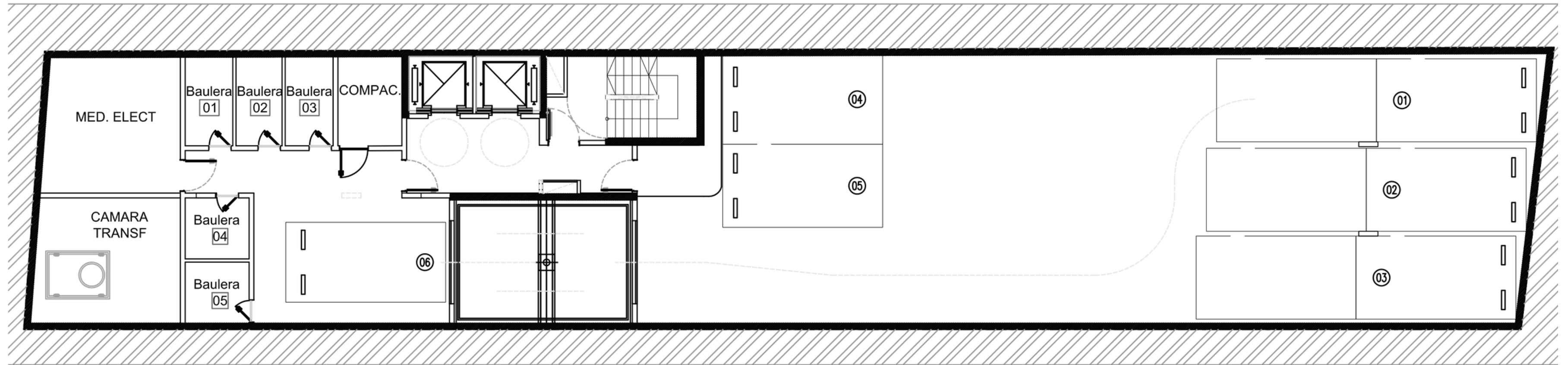
1er SUBSUELO (9 cocheras)
